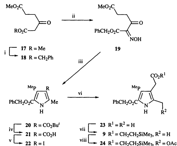
Scheme 3 Reagents: i, \text{PhCH}_2\text{OH} , heat; ii, \text{NaNO}_2 , \text{AcOH} ; iii, \text{MeCOCH}_2\text{CO}_2\text{Bu}^t , \text{Zn} , \text{AcOH} ; iv, \text{CF}_3\text{CO}_2\text{H} ; v, \text{KI}_3 , \text{NaHCO}_3 ; vi, \text{OHCCO}_2\text{H} , \text{HI} , \text{H}_3\text{PO}_2 , \text{Ac}_2\text{O} ; vii, (\text{COCl})_2 then \text{Me}_3\text{SiCH}_2\text{CH}_2\text{OH} ; viii, \text{SO}_2\text{Cl}_2 then \text{NaOAc} , \text{AcOH}
